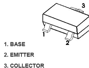
SOT-23
